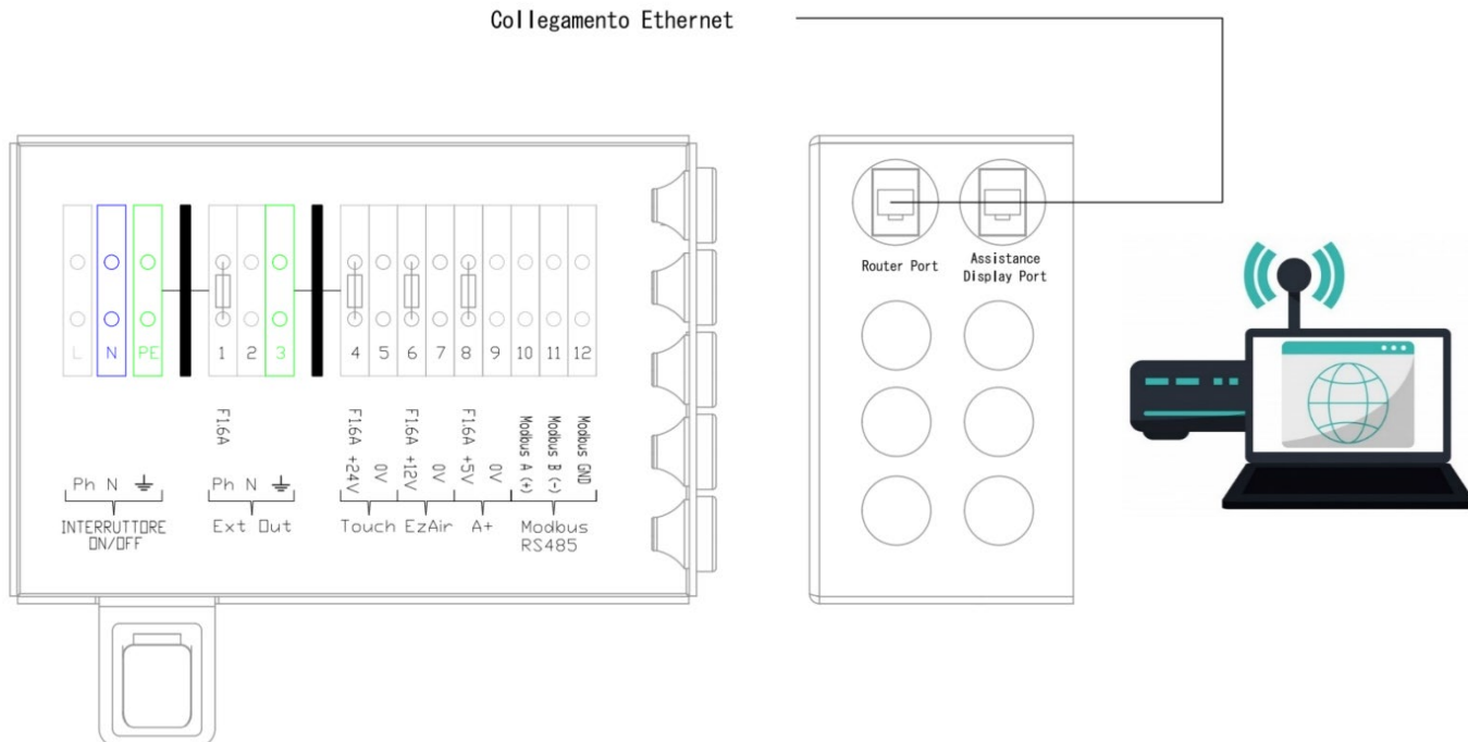
Collegamento Ethernet
